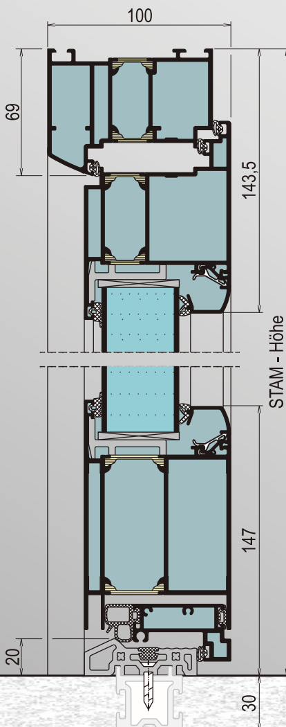
Rahmenbautiefe von 90 mm Zusammenbautiefe von 100 mm
